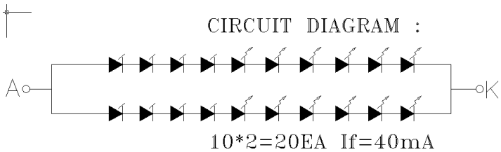
Fig.2*Schematics drawing of lighting（绘制照明图 图.2）
